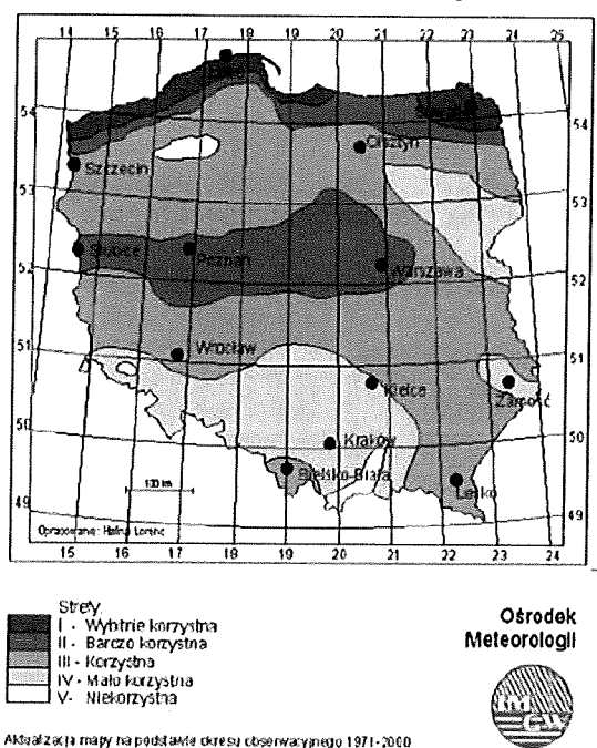
Rysunek 7 Zasoby energii wiatrowej w Polsce
