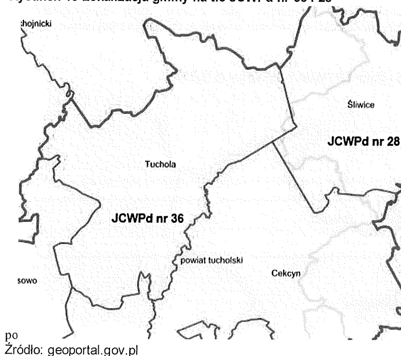
Rysunek 10 Lokalizacja gminy na tle JCWPd nr 36 i 28
