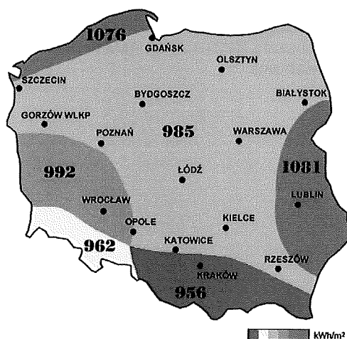
Rysunek 8 Usłonecznienie w Polsce w kWh/m 2
