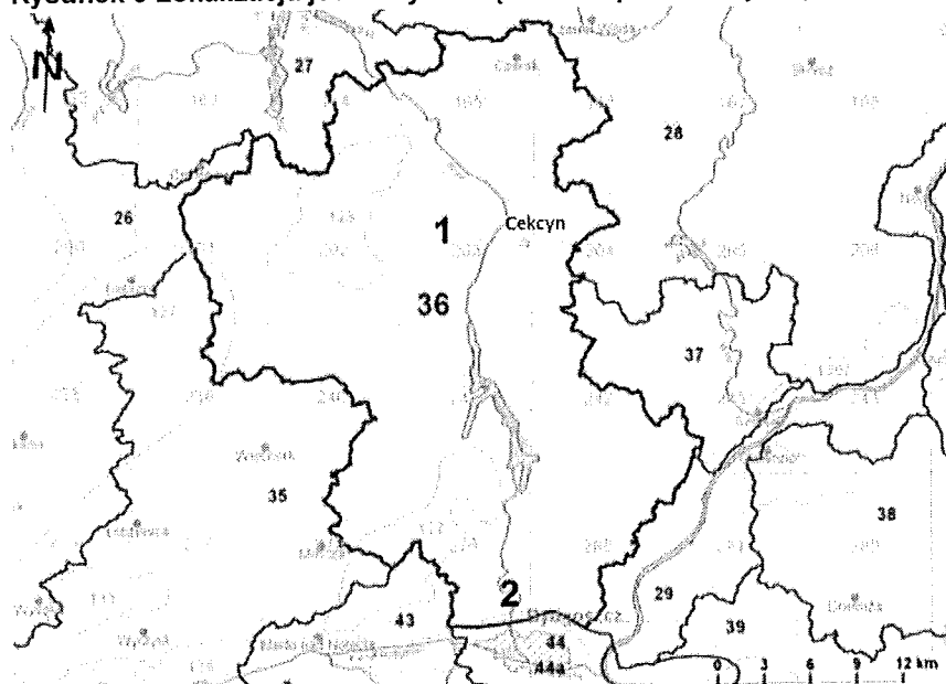
Rysunek 6 Lokalizacja jednolitych części wód podziemnych (JCWPd nr 36, 37 i 28)
